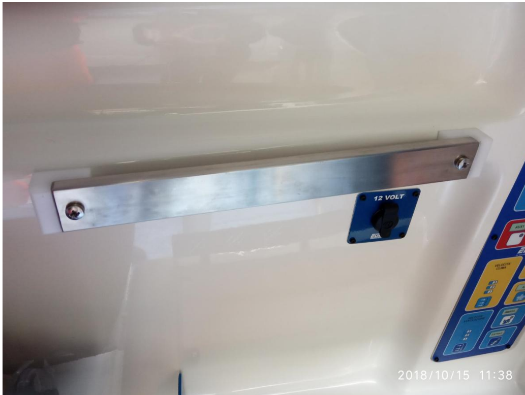
Figura 2: Dettaglio della barra DIN dell'ambulanza a cui il ventilatore d'emergenza (lotto 01) dovrà essere ancorato saldamente.
