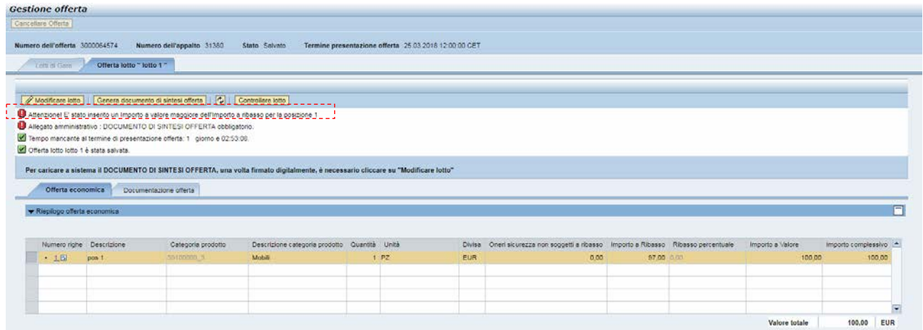
Figura 23 – Offerta economica superiore all’importo a ribasso
