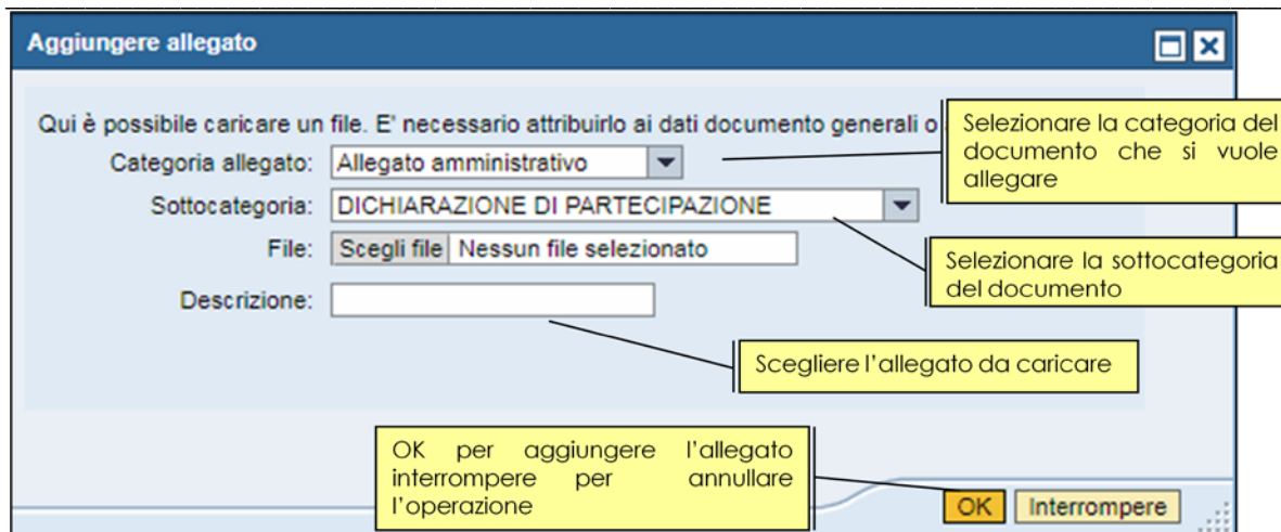
Figura 28 – Documentazione da allegare all’offerta telematica
